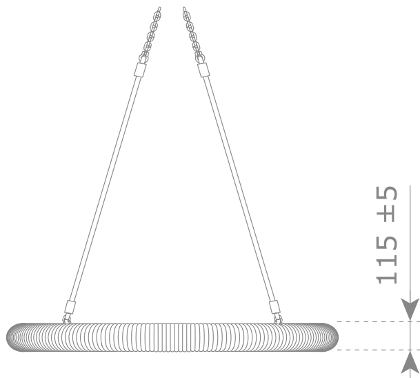
ALÇADO LATERAL SIDE VIEW
