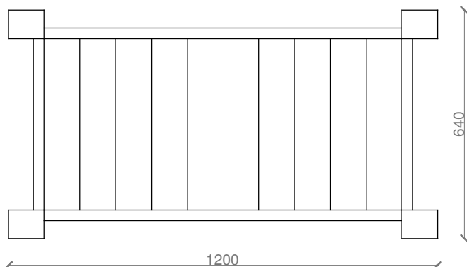
PLANTA
