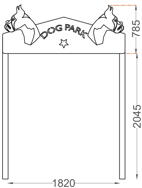
ALÇADO LATERAL SIDE VIEW
