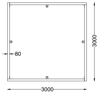
PLANTA PLAN
