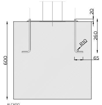
ALÇADO
