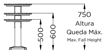
ALÇADO LATERAL SIDE VIEW
