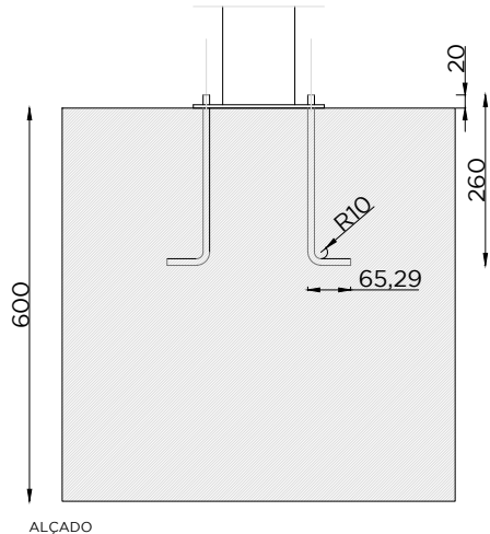
ALÇADO
