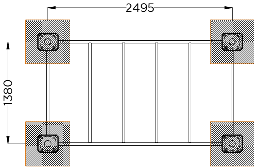
PLANTA . ESQUEMA DE FIXAÇÃO PLAN . INSTALLATION PLAN
