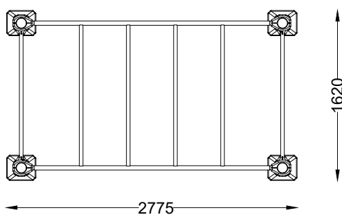
PLANTA PLAN
