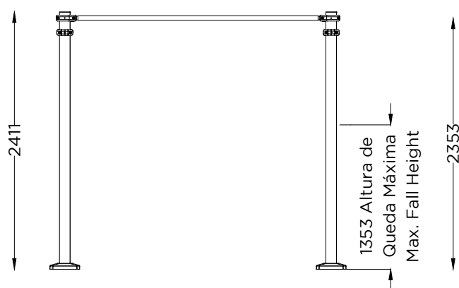
ALÇADO LATERAL SIDE VIEW
