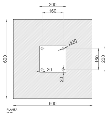
PLANTA PLAN
