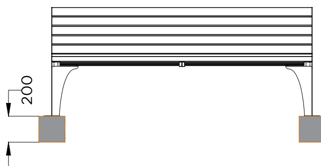
ALÇADO FRONTAL . ESQUEMA DE FIXAÇÃO FRONT VIEW . INSTALLATION PLAN
