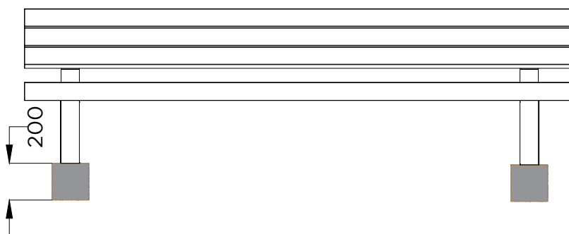
ALÇADO FRONTAL . ESQUEMA DE FIXAÇÃO FRONT VIEW . INSTALLATION PLAN
