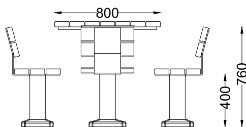
ALÇADO FRONTAL FRONT VIEW
