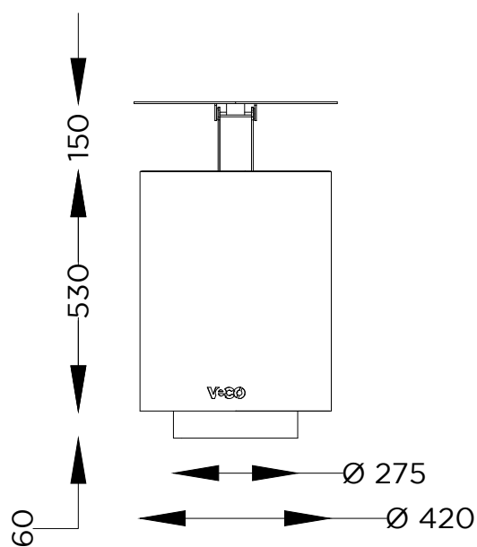
ALÇADO FRONTAL FRONT VIEW
