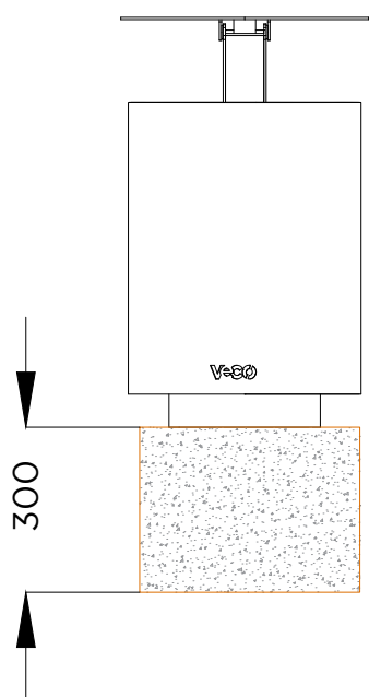
ALÇADO FRONTAL . ESQUEMA DE FIXAÇÃO FRONT VIEW . INSTALLATION PLAN
