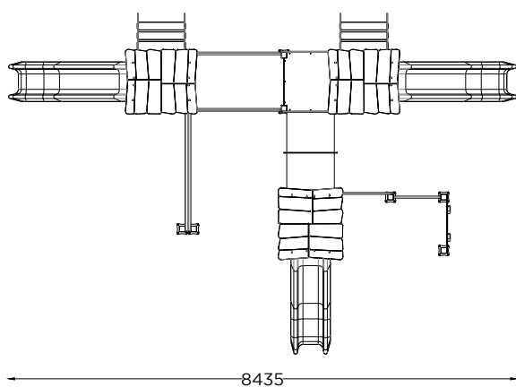
PLANTA PLAN
