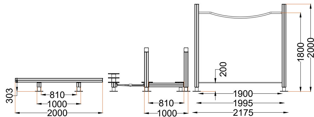
ALÇADO FRONTAL FRONT VIEW
