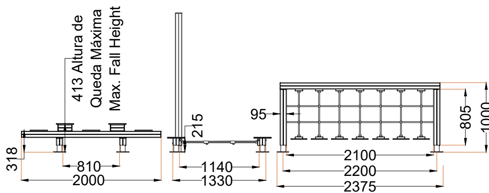
ALÇADO LATERAL SIDE VIEW
