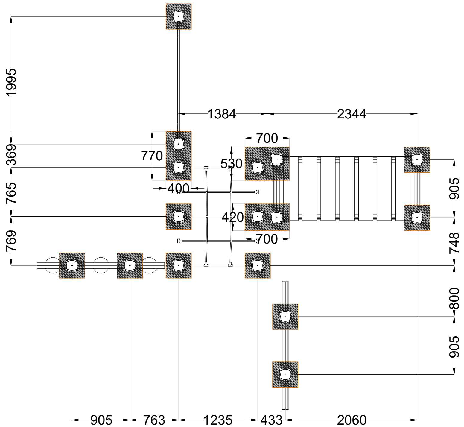
PLANTA . ESQUEMA DE FIXAÇÃO PLAN . INSTALLATION PLAN
