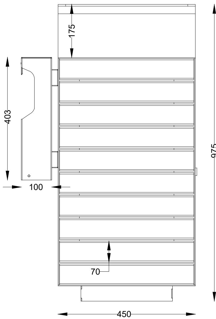
ALÇADO FRONTAL FRONT VIEW
