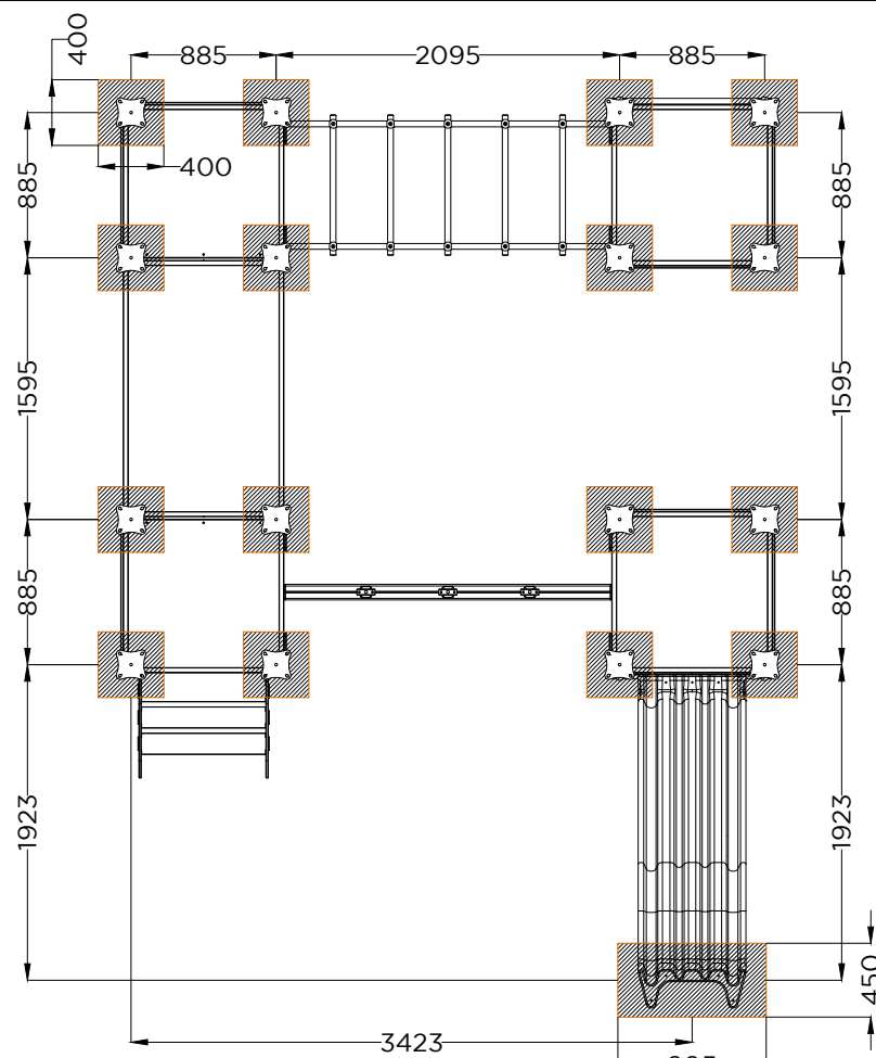
PLANTA . ESQUEMA DE FIXAÇÃO PLAN . INSTALLATION PLAN
