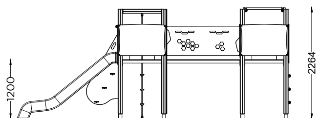
ALÇADO LATERAL SIDE VIEW
