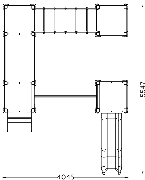
PLANTA PLAN
