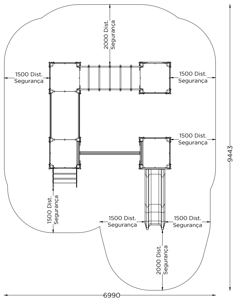
PLANTA - ESPAÇO DE SEGURANÇA NECESSÁRIO PLAN - SAFETY SPACE REQUIRED
