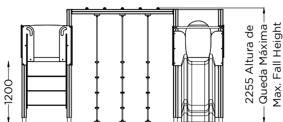
ALÇADO FRONTAL FRONT VIEW
