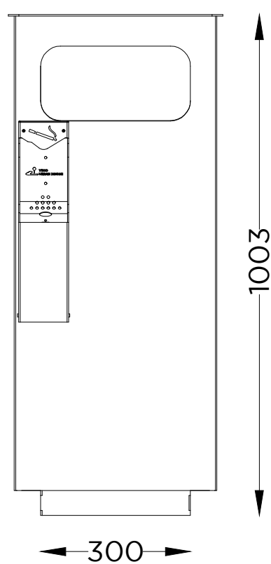
ALÇADO LATERAL SIDE VIEW
