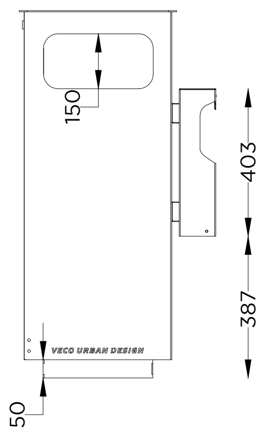
ALÇADO FRONTAL FRONT VIEW
