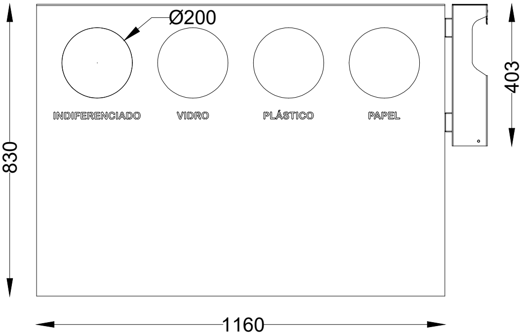
ALÇADO FRONTAL FRONT VIEW
