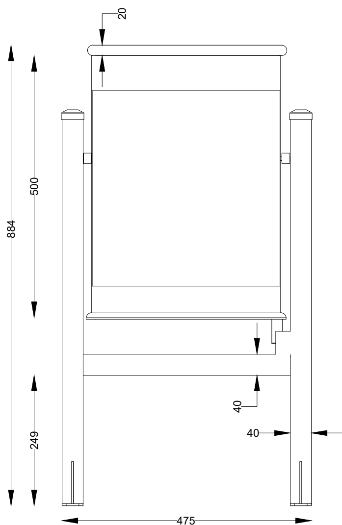
ALÇADO LATERAL SIDE VIEW
