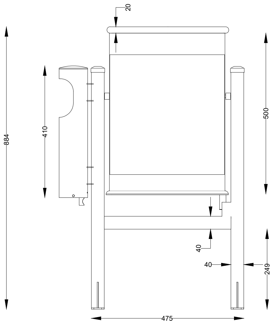
ALÇADO LATERAL SIDE VIEW
