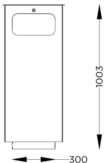
ALÇADO LATERAL SIDE VIEW
