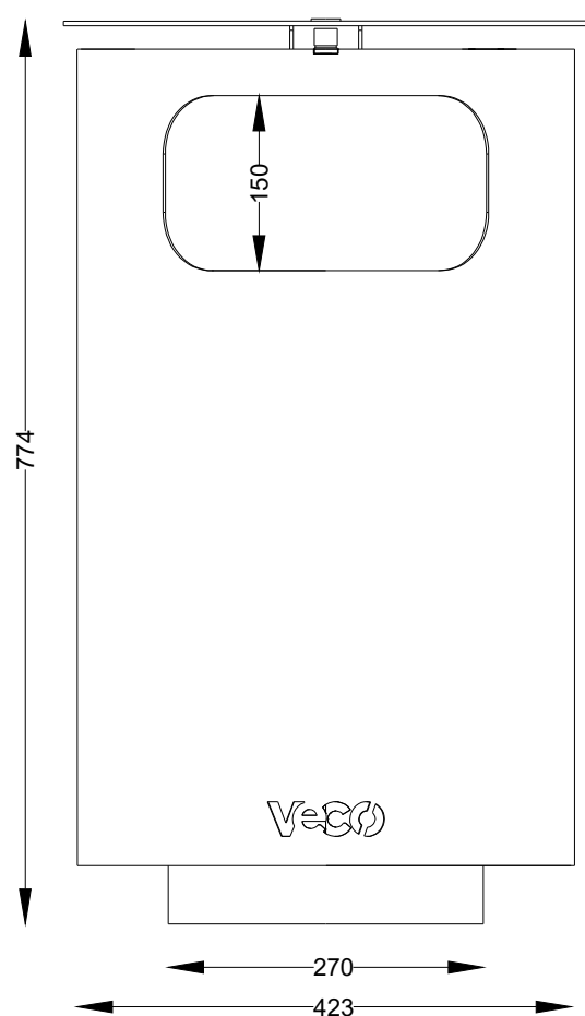
ALÇADO FRONTAL FRONT VIEW
