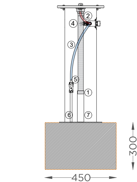
ALÇADO
