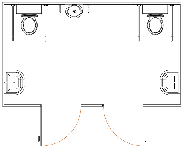
PLANTA . PLAN .
