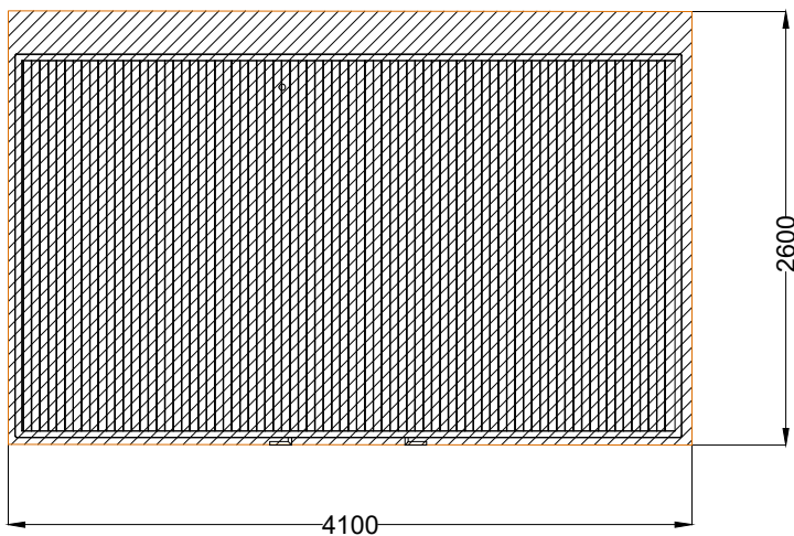
PLANTA . ESQUEMA DE FIXAÇÃO PLAN . INSTALLATION PLAN
