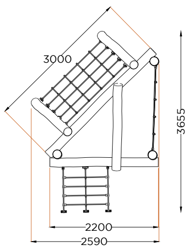
PLANTA - ESPAÇO DE SEGURANÇA NECESSÁRIO PLAN - SAFETY SPACE REQUIRED
