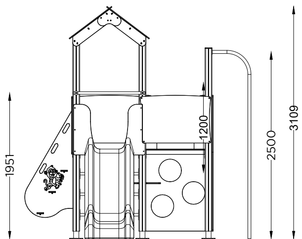
ALÇADO FRONTAL FRONT VIEW
