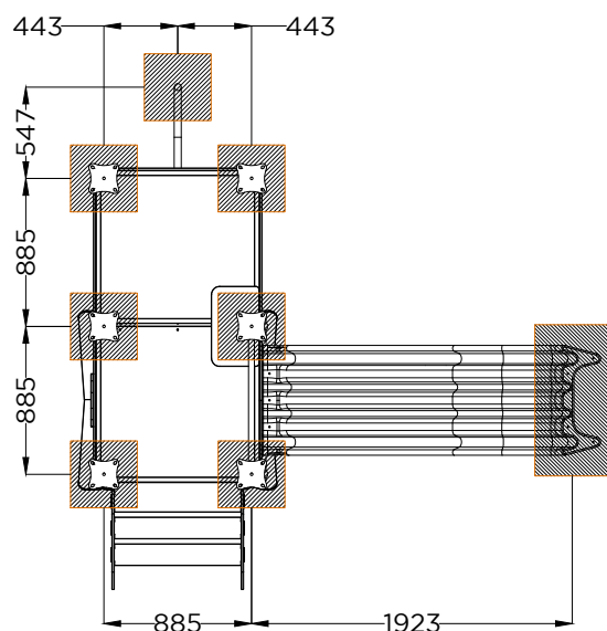
PLANTA . ESQUEMA DE FIXAÇÃO PLAN . INSTALLATION PLAN
