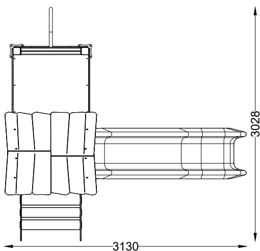
PLANTA PLAN
