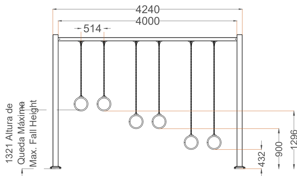
ALÇADO FRONTAL FRONT VIEW
