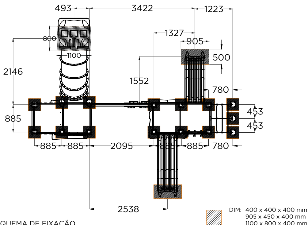
PLANTA . ESQUEMA DE FIXAÇÃO PLAN . INSTALLATION PLAN
