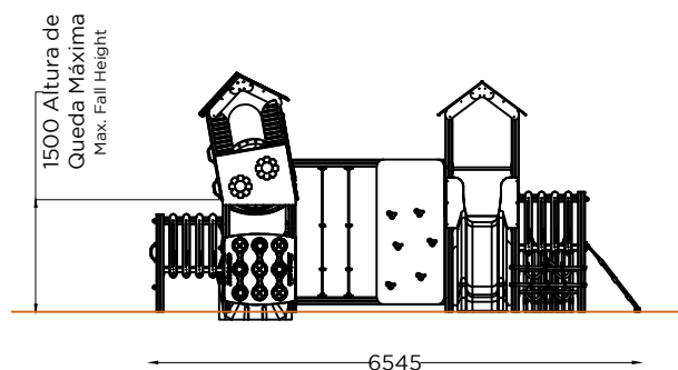
ALÇADO LATERAL SIDE VIEW
