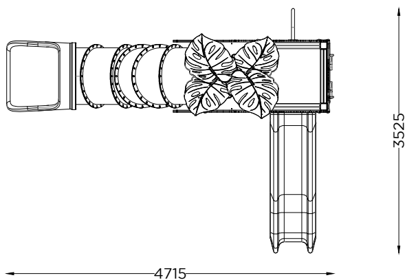
PLANTA PLAN
