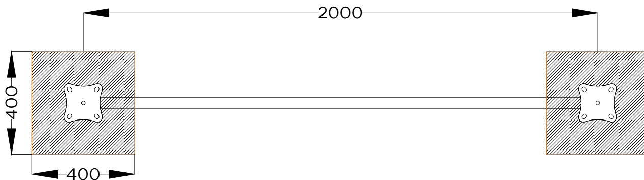
PLANTA - ESPAÇO DE SEGURANÇA NECESSÁRIO PLAN - SAFETY SPACE REQUIRED
