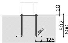
ALÇADO FRONTAL FRONT VIEW
