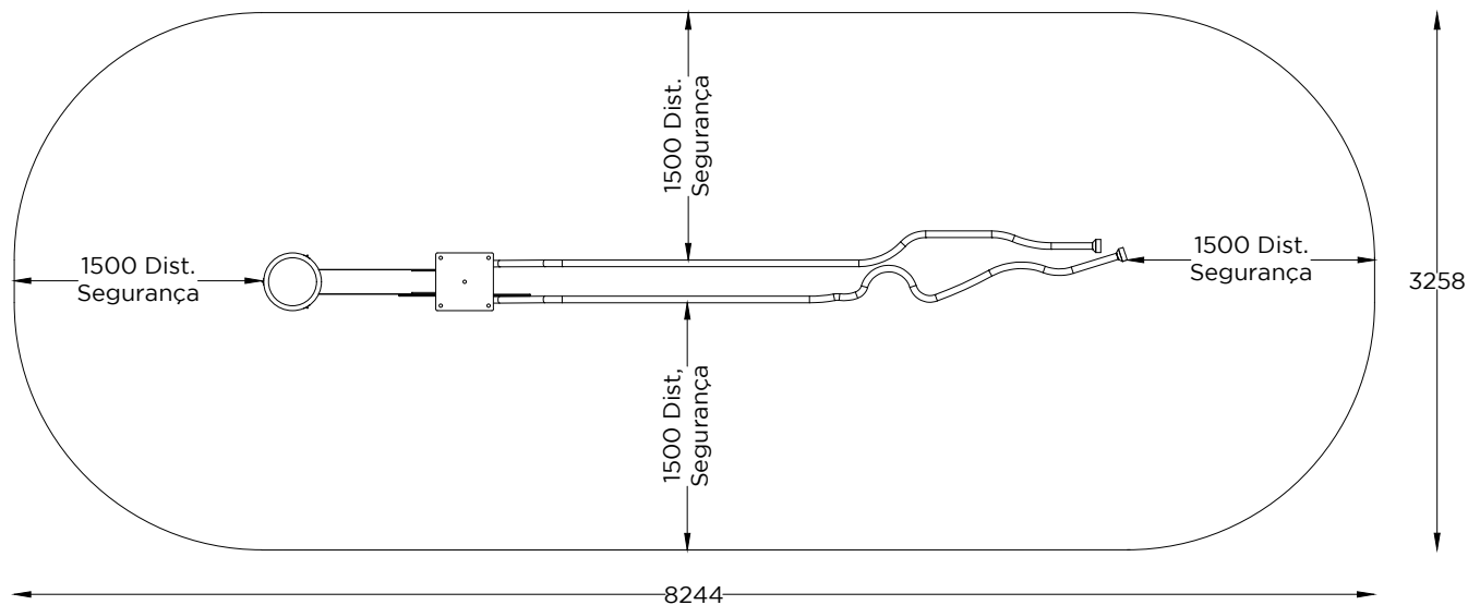
PLANTA - ESPAÇO DE SEGURANÇA NECESSÁRIO PLAN - SAFETY SPACE REQUIRED
