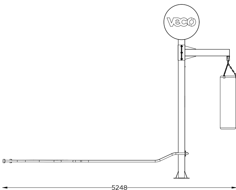
ALÇADO LATERAL SIDE VIEW
