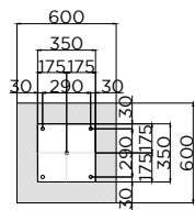
PLANTA PLAN
