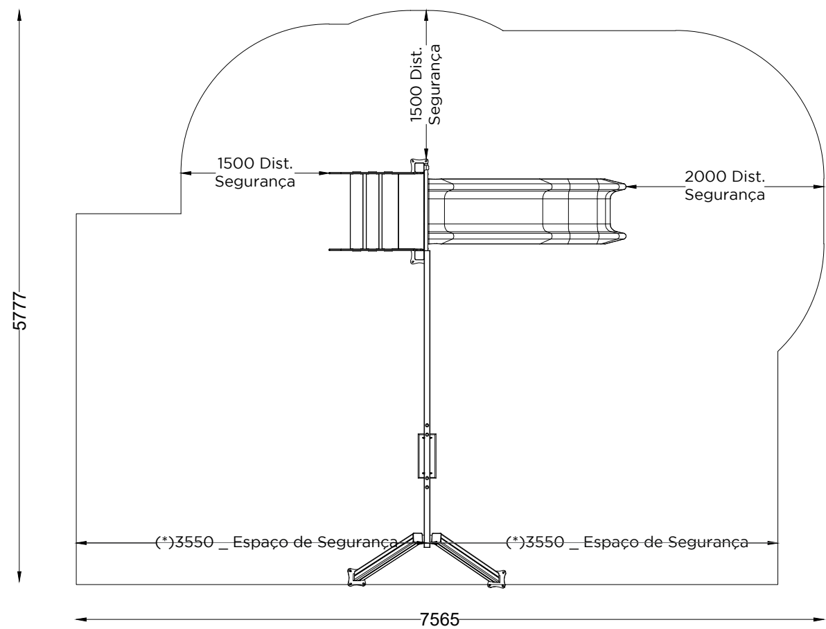
PLANTA - ESPAÇO DE SEGURANÇA NECESSÁRIO PLAN - SAFETY SPACE REQUIRED
