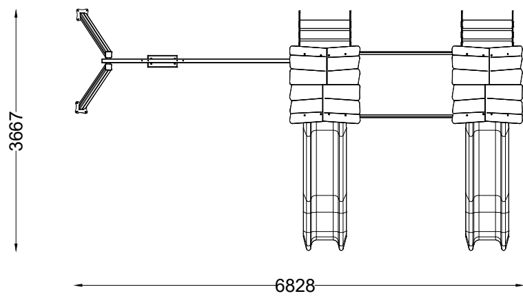
PLANTA PLAN
