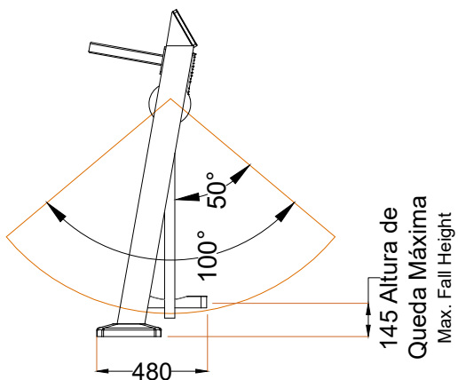
ALÇADO LATERAL SIDE VIEW
