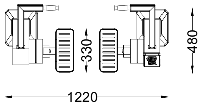
PLANTA PLAN
