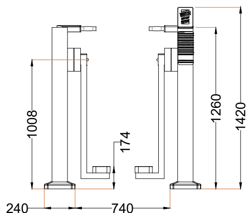
ALÇADO FRONTAL FRONT VIEW
