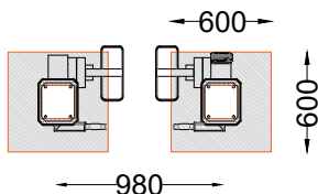
PLANTA . ESQUEMA DE FIXAÇÃO PLAN . INSTALLATION PLAN
