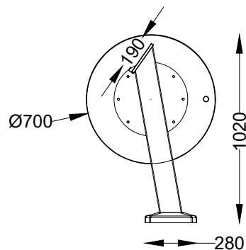
ALÇADO FRONTAL FRONT VIEW
