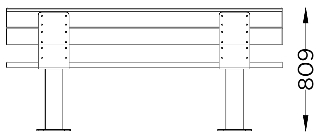
ALÇADO LATERAL SIDE VIEW
