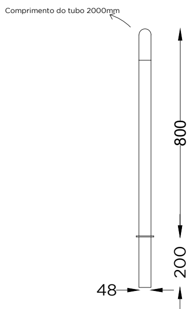
ALÇADO LATERAL SIDE VIEW
