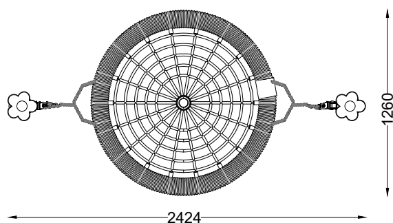
PLANTA PLAN
