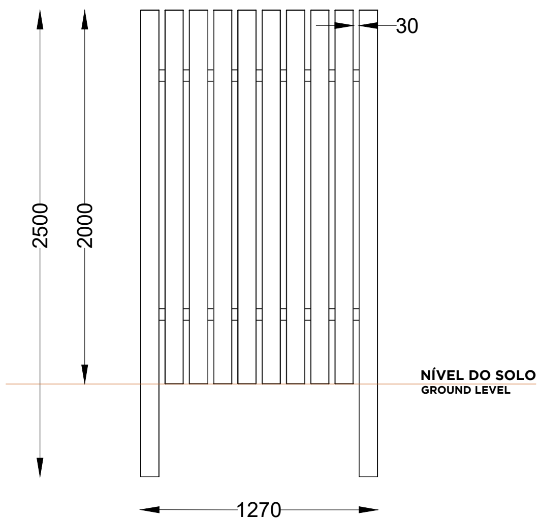
ALÇADO FRONTAL FRONT VIEW
