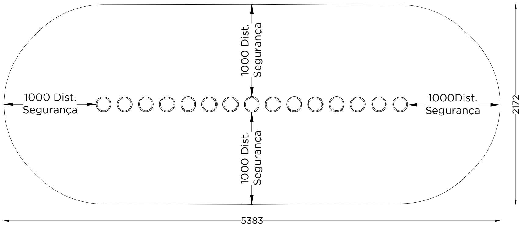
PLANTA - ESPAÇO DE SEGURANÇA NECESSÁRIO PLAN - SAFETY SPACE REQUIRED
