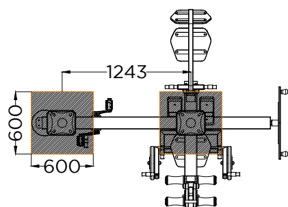
PLANTA . ESQUEMA DE FIXAÇÃO PLAN . INSTALLATION PLAN
