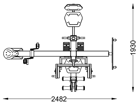
PLANTA PLAN
