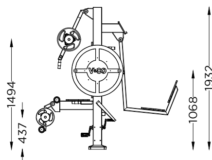
ALÇADO LATERAL SIDE VIEW
