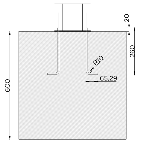
ALÇADO
