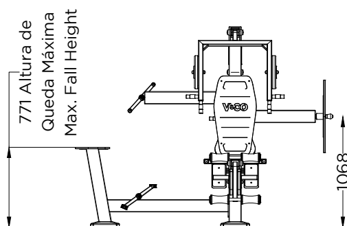
ALÇADO FRONTAL FRONT VIEW
