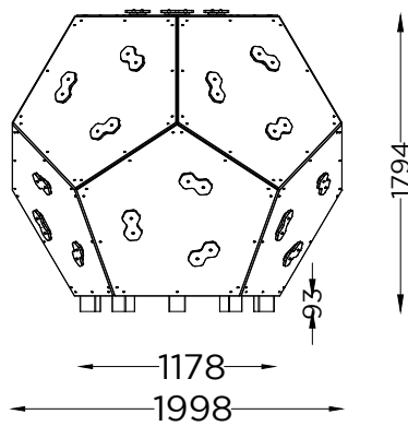
ALÇADO FRONTAL FRONT VIEW
