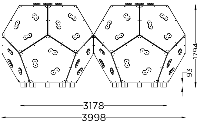
ALÇADO FRONTAL FRONT VIEW
