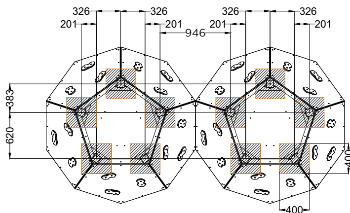
PLANTA . ESQUEMA DE FIXAÇÃO PLAN . INSTALLATION PLAN
