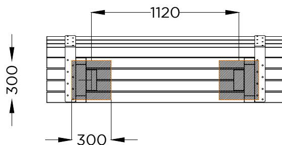
PLANTA . ESQUEMA DE FIXAÇÃO PLAN . INSTALLATION PLAN
