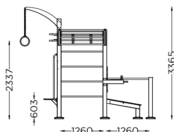
ALÇADO LATERAL SIDE VIEW
