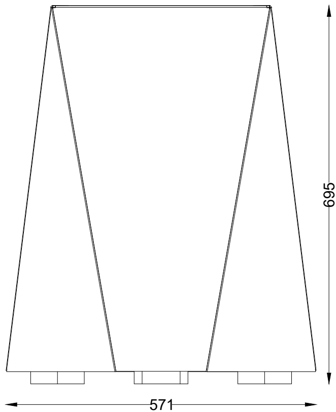
ALÇADO LATERAL SIDE VIEW
