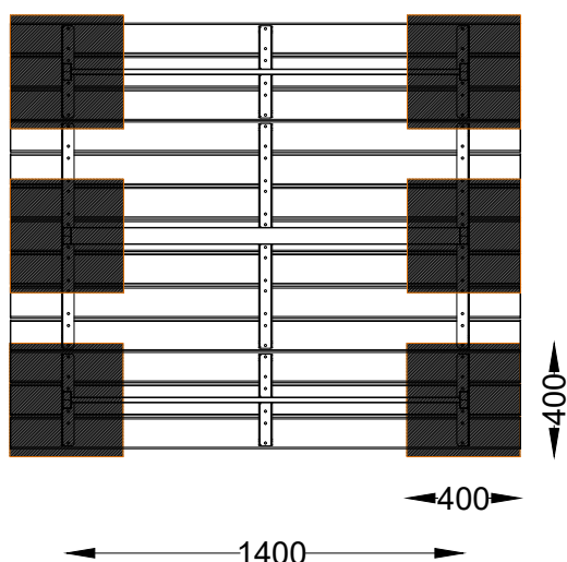
PLANTA . ESQUEMA DE FIXAÇÃO PLAN . INSTALLATION PLAN
