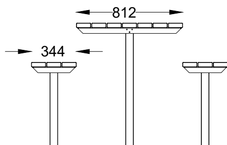
ALÇADO LATERAL SIDE VIEW
