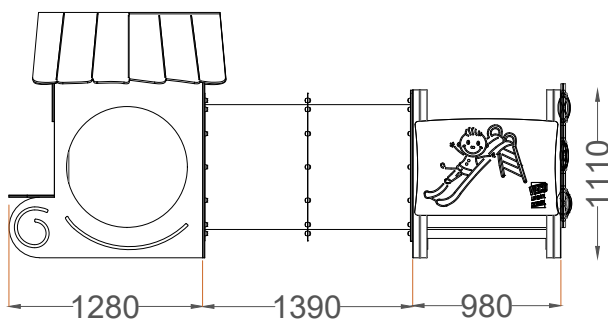
ALÇADO FRONTAL FRONT VIEW
