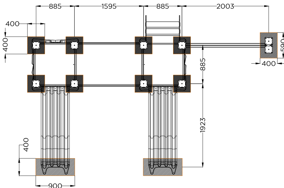
PLANTA . ESQUEMA DE FIXAÇÃO PLAN . INSTALLATION PLAN
