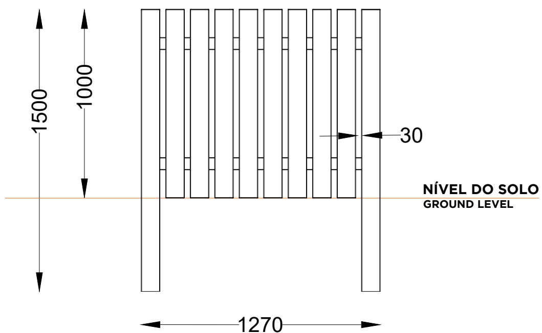
ALÇADO FRONTAL FRONT VIEW
